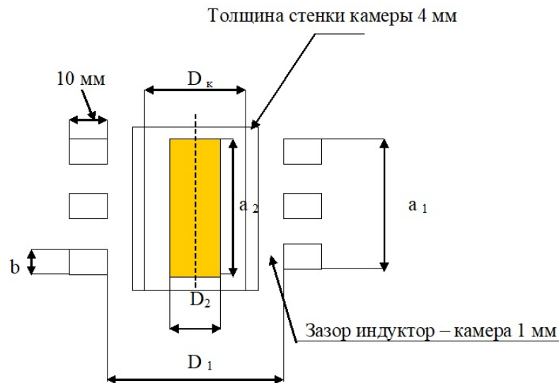
Рисунок 1 – Расчётная схема системы индуктор – плазма
