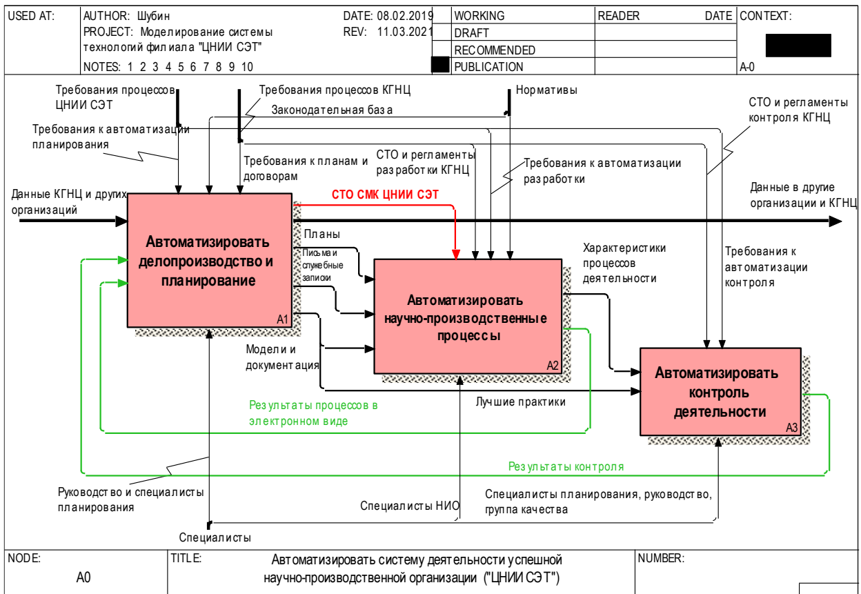
Рисунок 6 – Диаграмма модели целевого состояния системы классов технологий примера НПОР
